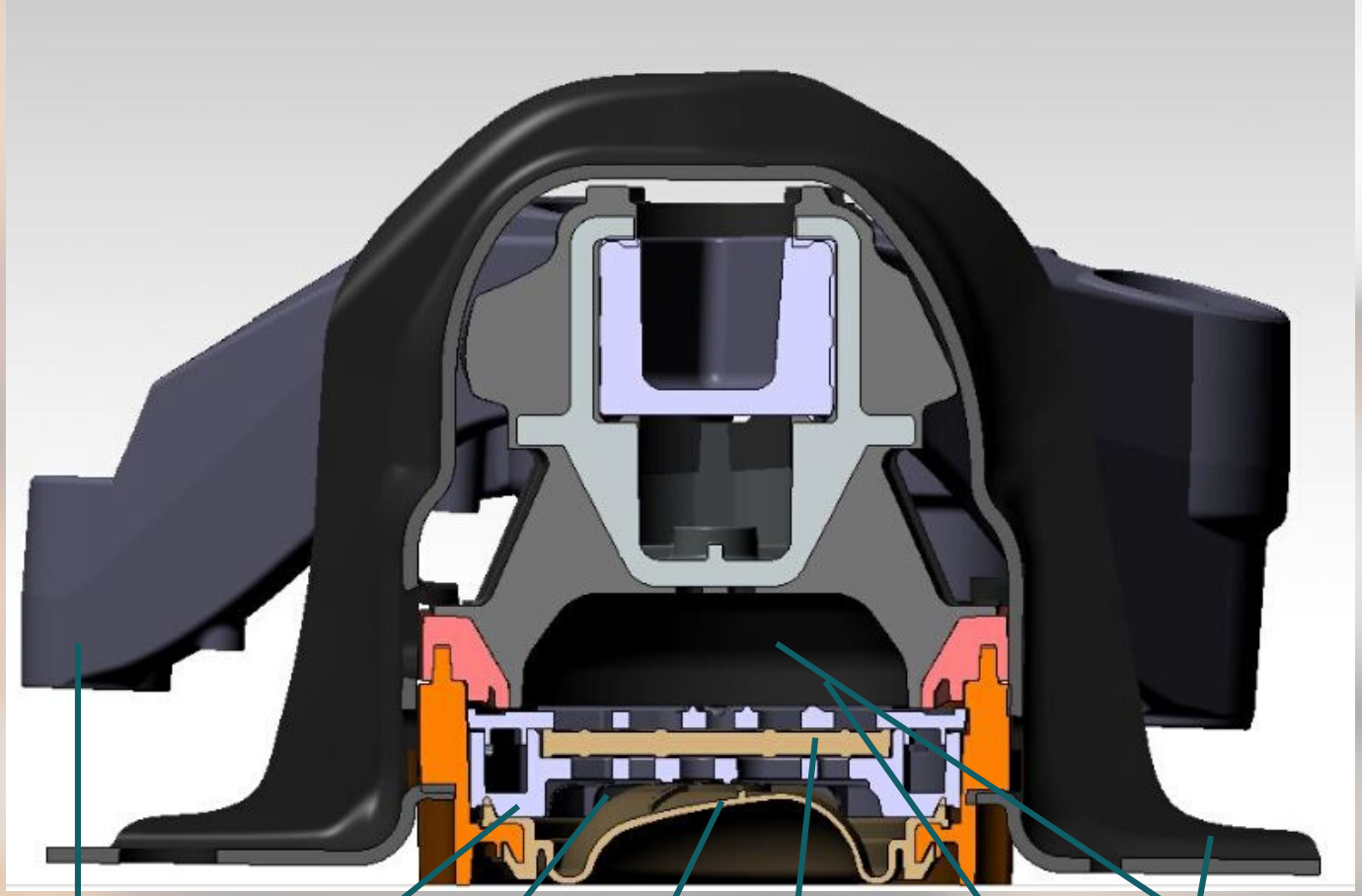
Alüminyum Kol (Motor Tarafı) Alt süzgeç Alt oda Diyafram Süzgeç Contası Üst oda Liquid Gövde Sacı (Şasi Tarafı)
